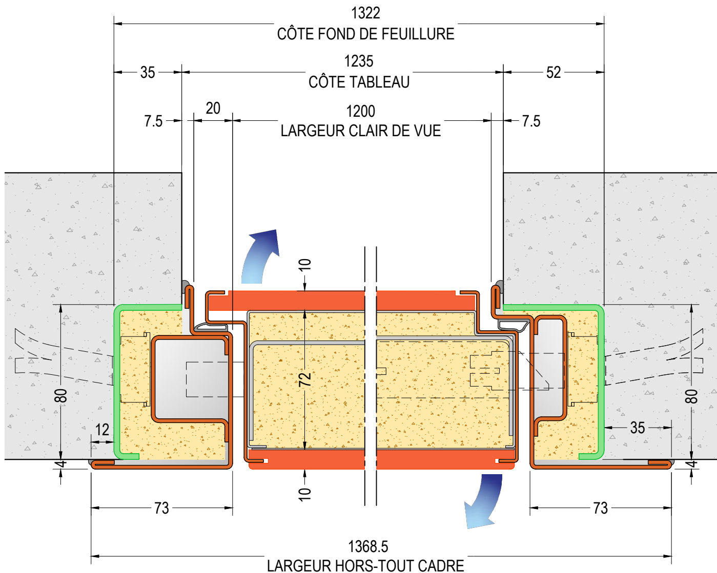
COUPE HORIZONTALE DE LA PORTE MODÈLE "A" réf. PORTE L=1200(900+300)
