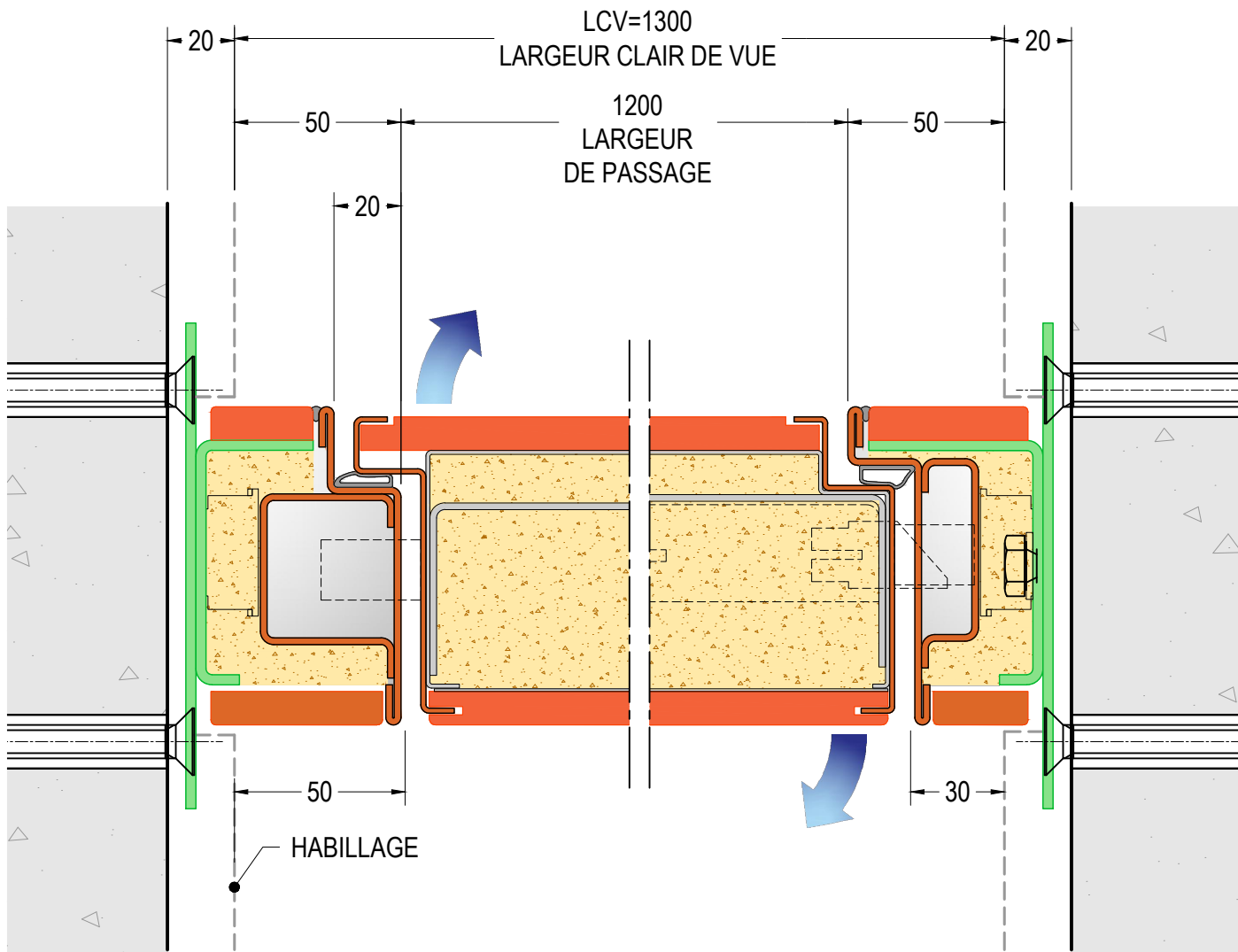
COUPE HORIZONTALE DE LA PORTE MODÈLE "A" réf. PORTE L=1200(900+300)
