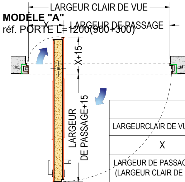
CALCULER LA LARGEUR DE PASSAGE
