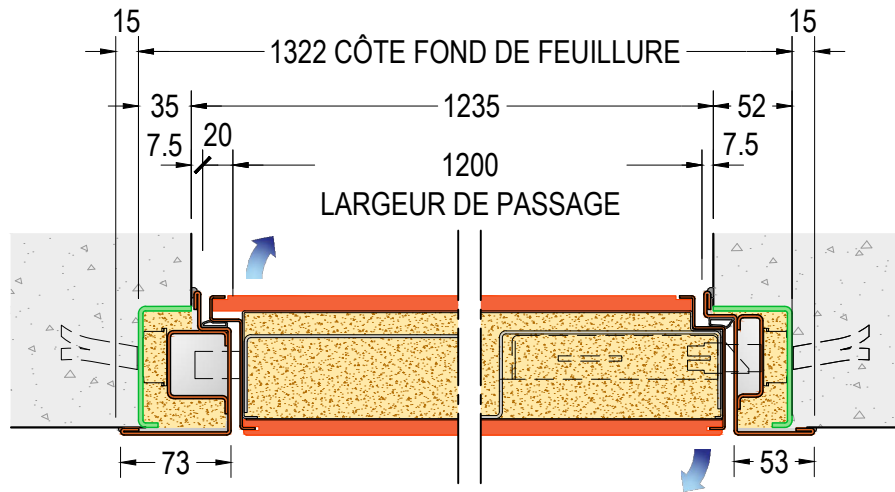
COUPE HORIZONTALE DE LA PORTE - MODÈLE "B" réf. PORTE L=1200 - LARGEUR CLAIR DE VUE LCV=1200
