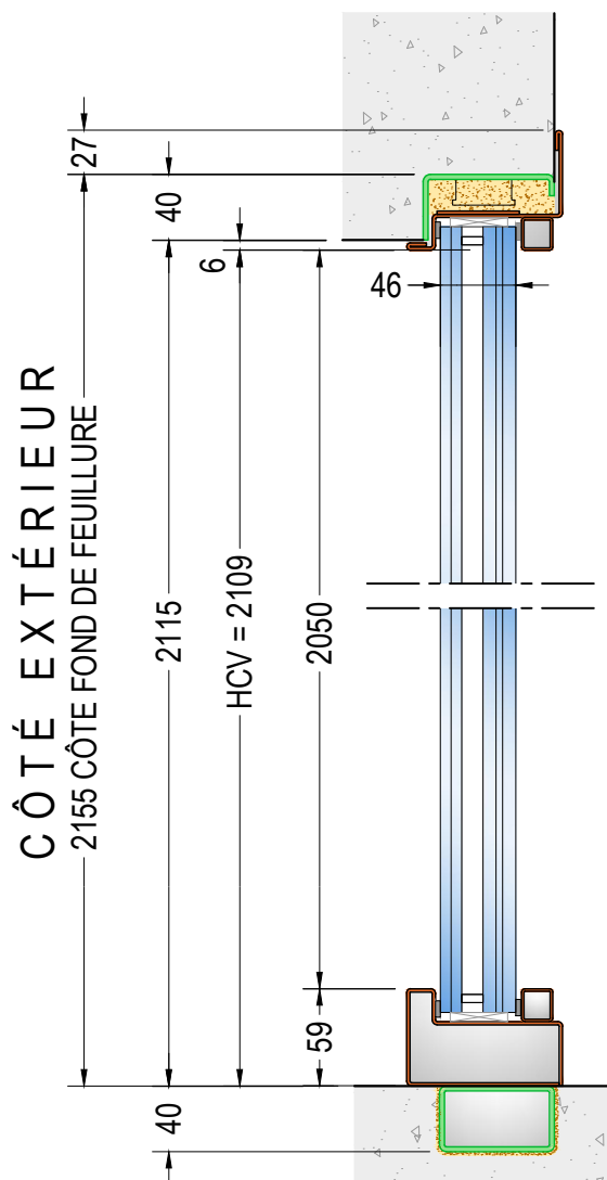
COUPE VERTICALE DES FIXES LATÉRAUX VITRÉS - MODÈLES "F-G-H" réf. PORTE H=2100 HAUTEUR CLAIR DE VUE HCV=2109
